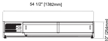
VTPSL-139 Front
