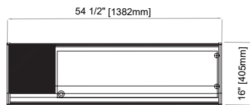
VTPSL-139 Top
